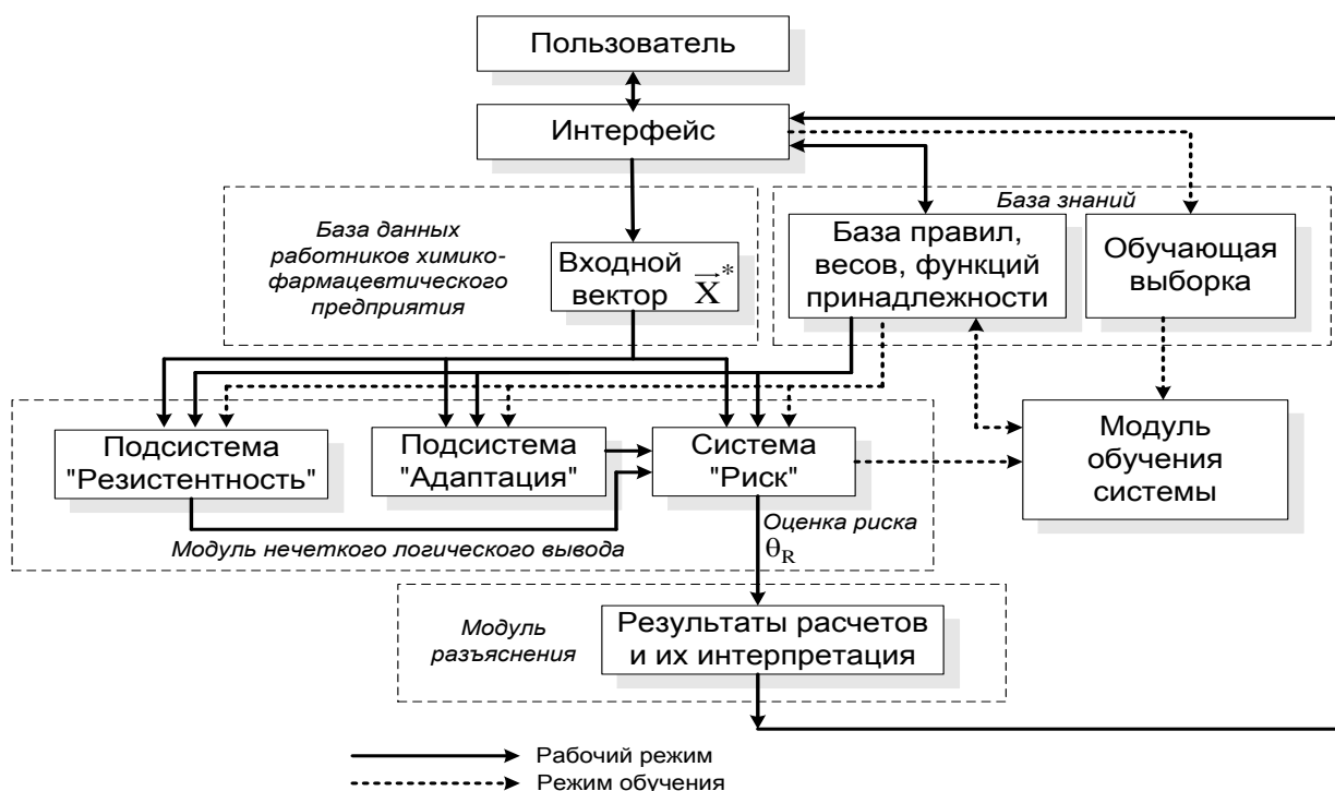
Рис. 2. Структурная схема дополненной НЭС оценки риска развития ПОЗ
