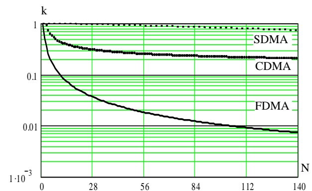
Рис. 2. Коэффициент использования частотного ресурса
