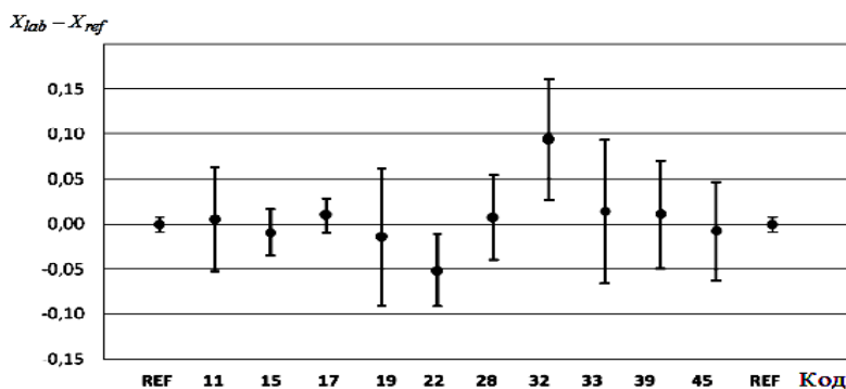
Рис. 2. Диаграмма результатов измерений при 0 °С
