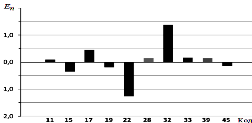
Рис. 3. Значения E_n при 0 °С
