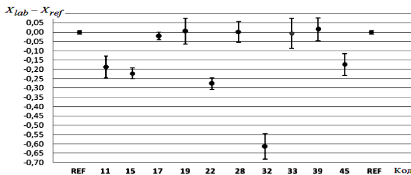
Рис. 4. Диаграмма результатов измерений при 100 °С
