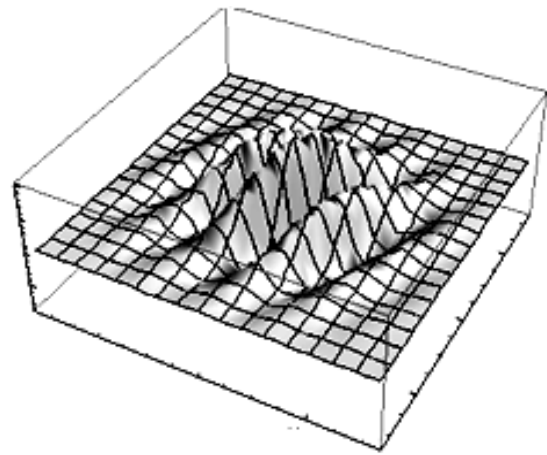
Рис. 4. Вейвлет Габора на плоскости
