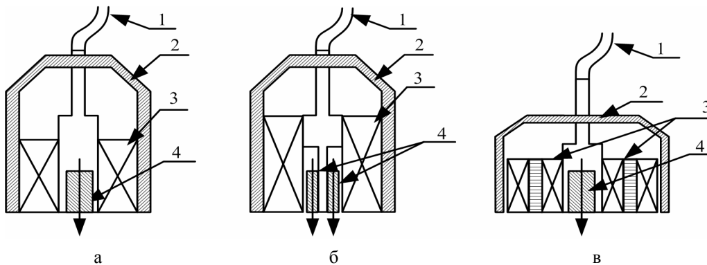
Рис. 3. Схеми вихрострумних перетворювачів: а – з одним магніторезистором в середині котушки збудження; б – з двома диференційно-включеними магніторезисторами в середині котушки збудження в – з одним магніторезистором та двома котушками (1 – екранований кабель, 2 – екранований корпус, 3 – котушка збудження, 4 – магніторезистор з позначеною віссю чутливості)
