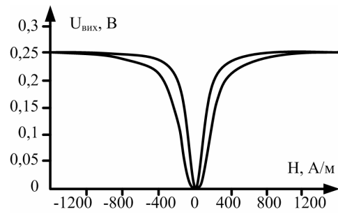
Рис. 2. Характеристика перетворення магніторезистора ААН002-02
