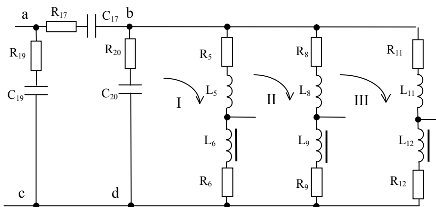
Рис. 6. Еквівалентна схема заміщення системи системи електропостачання
