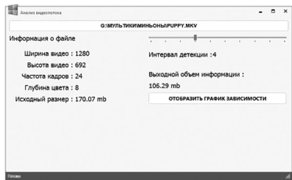
Рис. 2. Интерфейс модуля
