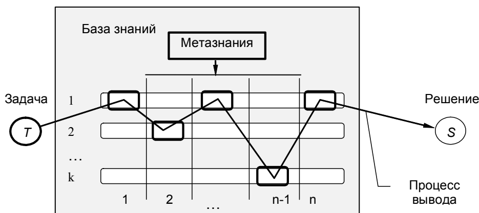
Рис. 3. Схема вывода на многоэкспертных знаниях
