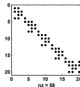
Рис. 7. Структура матрицы А
