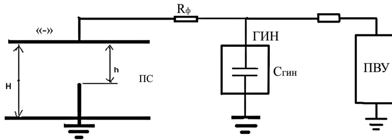
Рис. 2. Схема испытаний
