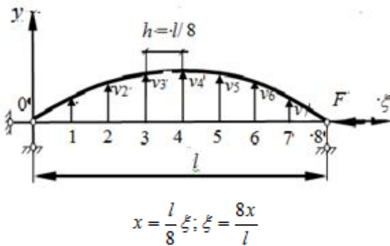
Рис. 2. Численный пример
