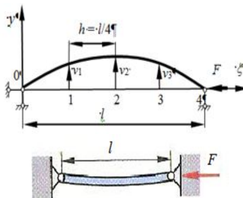
Рис. 1. Задача Эйлера
