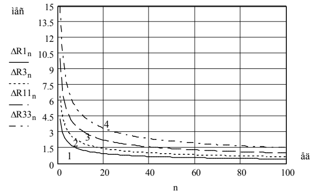
Рис. 4. Графики зависимостей величин ошибок определения среднего ресурса от n для нормального (график 1 при \gamma=0,8 ; график 2 при \gamma=0,9 ) и произвольного (график 3 при \gamma=0,8 ; график 4 при \gamma=0,9 ) законов распределения наработки до ресурсного отказа
