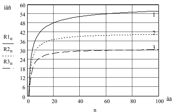
Рис. 3. Графики зависимостей уточнённой величины ОНДГ R_{ty}^{(H)}(\tau) от количества изделий при: 1) \gamma=0,8 , P(\tau)=1 , t=62 ; 2) \gamma=0,8 , P(\tau)=0,9 , t=62 ; 3) \gamma=0,8 , P(\tau)=0,8 , t=62
