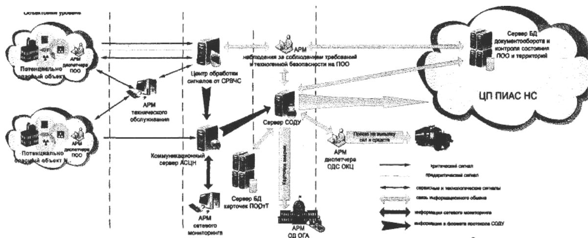
Рис. 2. Структура УІАС, яка пропонується
