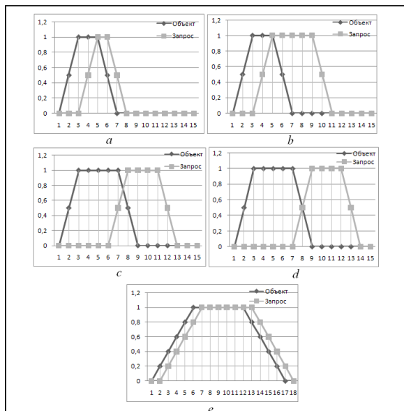
Рис. 4. Функции, в которых объект частично покрывает запрос: а – P=0,67; б – P=0,33; с – P=0,19; д – P=0,1; е – P=5
