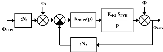
Рис. 2. Эквивалентная схема ИФАПЧ со смесителем и ДПКД в обратной связи и источниками шумов приведенным к двум источникам
