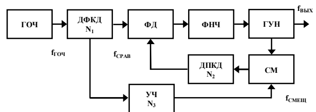
Рис. 1. Структурная схема однокольцевой ИФАПЧ со смесителем
