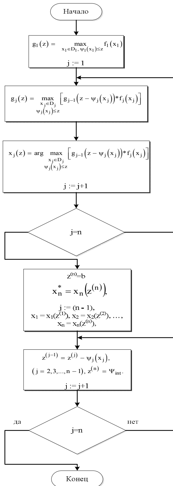
Рис. 5. Алгоритм метода динамического программирования
