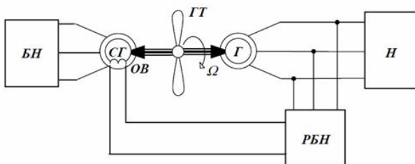
СГ – синхронний генератор; ОВ - обмотка збудження
