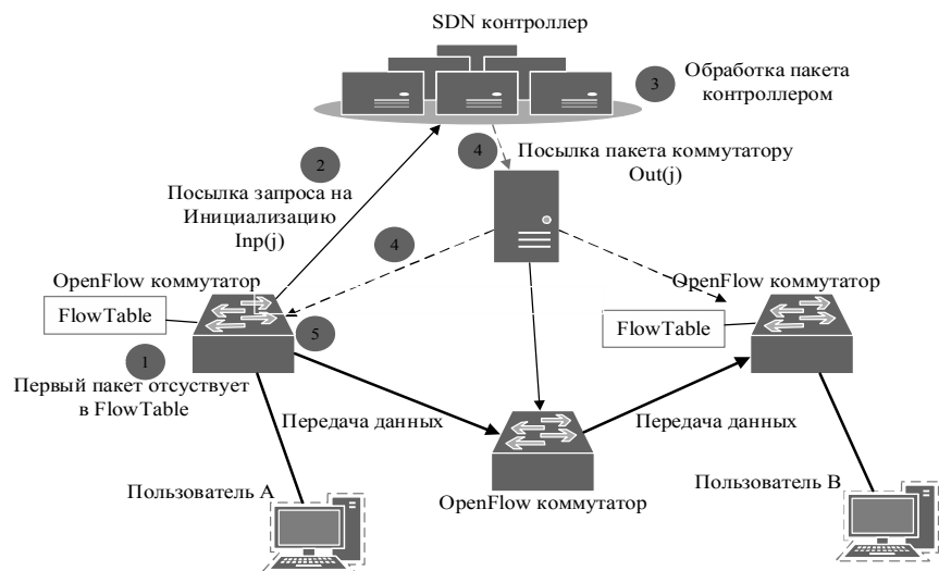
Рис. 2. Формування управляючого потоку в SDN
