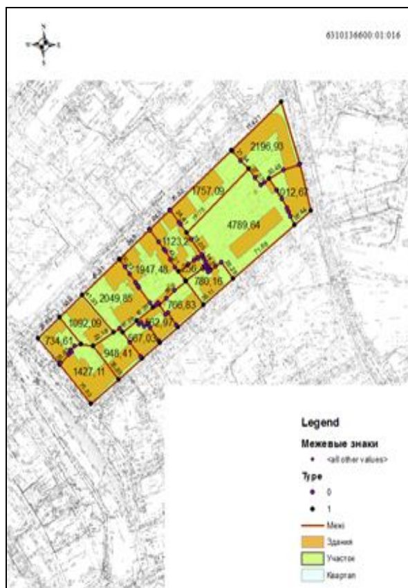
Рис. 6. Кадастровый план
