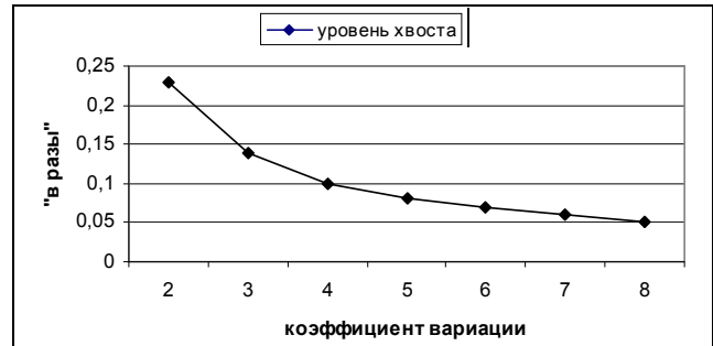
Рис. 3. Зависимость уровня хвоста гиперэкспоненциального распределения по отношению к распределению Парето
