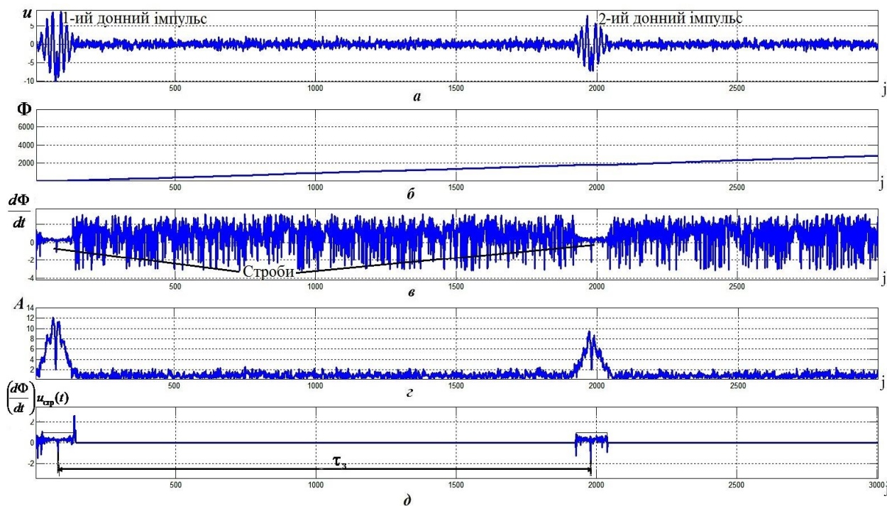
Рис. 3. Результати моделювання двошкального способу ультразвукової товщинометрії
