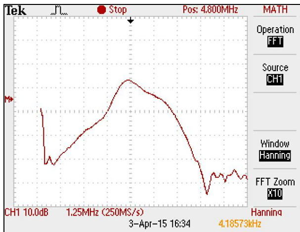
Рис. 5. АЧХ перетворювача П211-5-Р20
