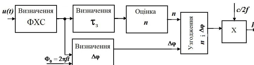
Рис. 1. Структурно-логічна схема двошкального методу ультразвукової лунаімпульсної товщинометрії
