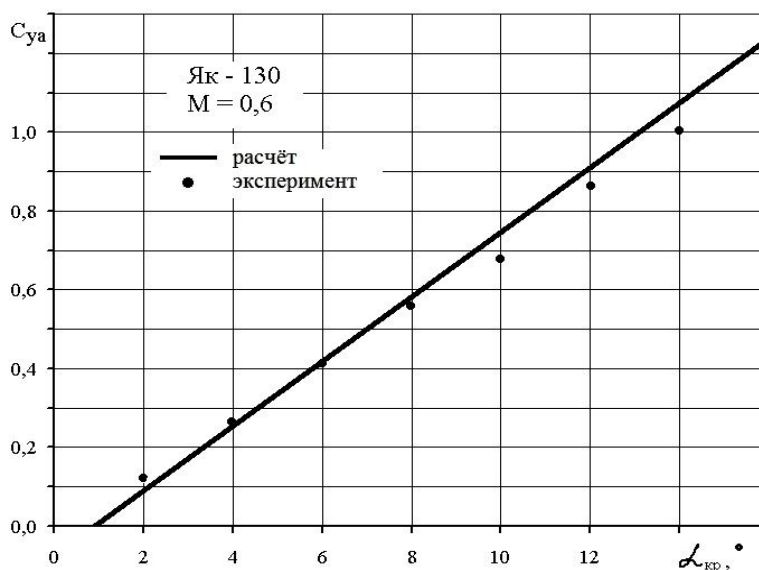
Рис. 2. Зависимости балансировочных значений C_{ya} самолета Як-130 от угла атаки
