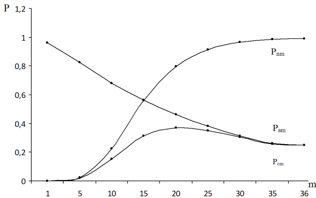
Рис. 4. Залежності ймовірностей безвідмовної роботи апаратних засобів ( P_{ам} ), програмного забезпечення ( P_{пм} ) і системи в цілому ( P_{см} ) від часу експлуатації
