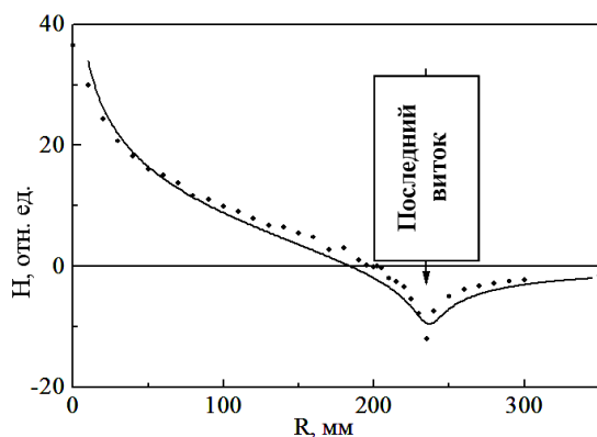
Рис. 11. Измеренная (точки) и теоретическая (линия) конфигурация магнитного поля плоской спирали
