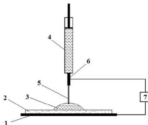
Рис. 1. Експериментальна установка для отримання зображень газорозрядного випромінювання рідиннофазних об'єктів
