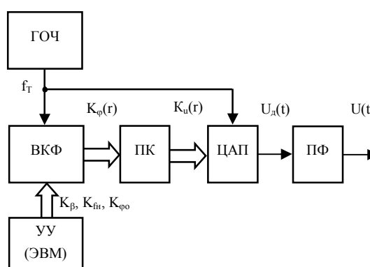
Рис. 1. Структурная схема формирователя ЛЧМ сигнала методом прямого цифрового синтеза
