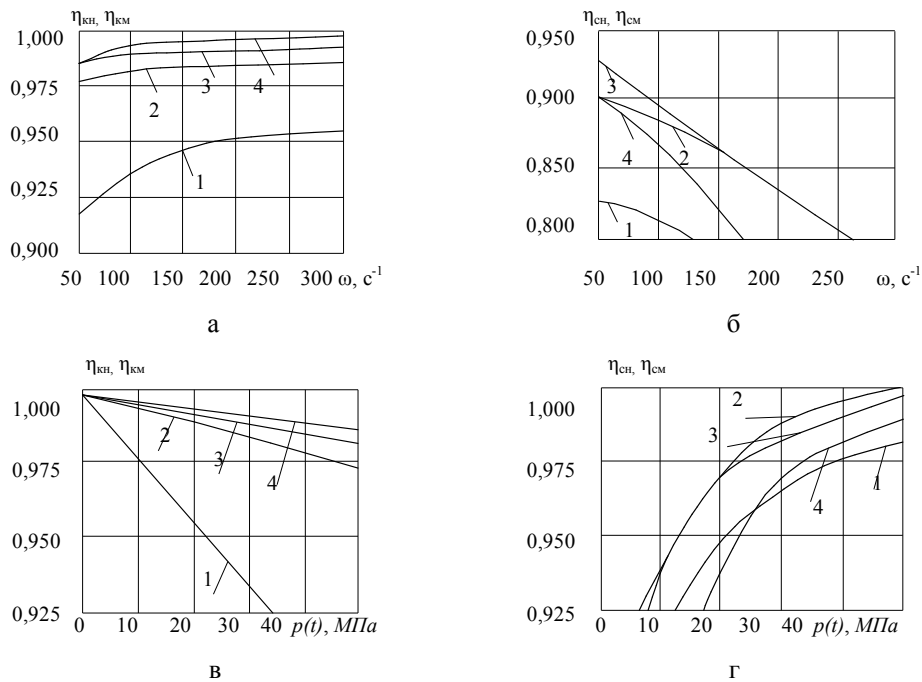
Рис. 3. Кінематичний (а, в) та силовий (б, г) к.к.д. аксіально-поршневих гідромашин типу «Зауер» при p = 20 МПа (а, б) або \omega = 300 с -1 (в, г): 1 – \eta_{\text{кн}} при \beta = 0,3 ; 2 – \eta_{\text{кн}} при \beta = 0,7 ; 3 – \eta_{\text{кн}} при \beta = 1 ; 4 – \eta_{\text{см}}
