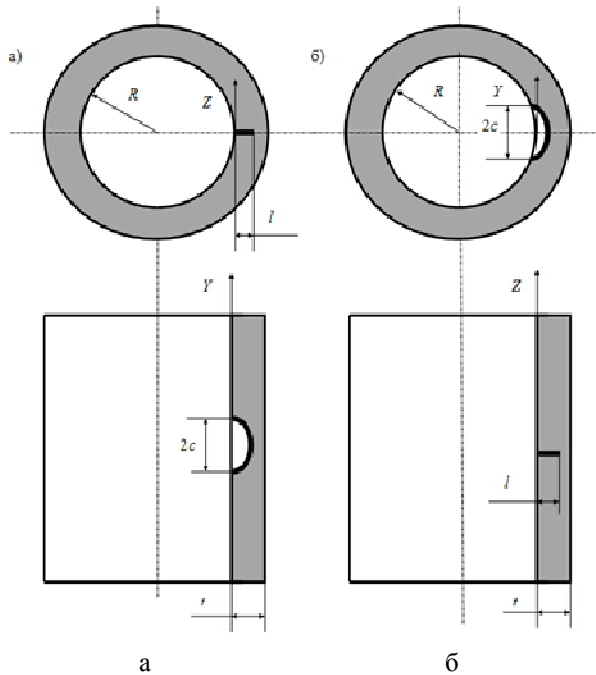
Рис. 2. Схема елемента з тріщиною на поверхні з кривизною: а – уздовж осі Z; б – уздовж осі Y
