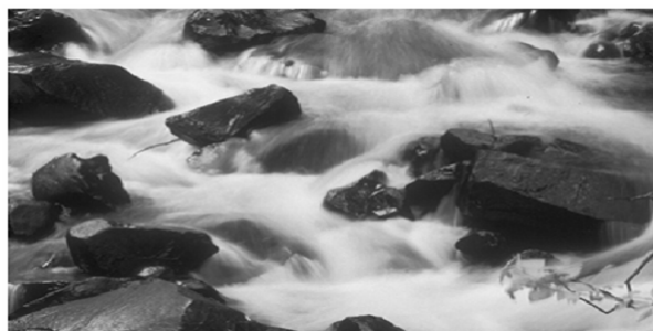
Рис. 2. Вихідне зображення [12]
