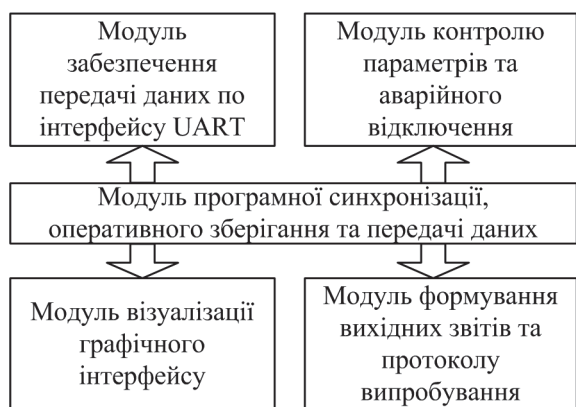
Рис. 9. Структура спеціалізованого програмного забезпечення комп'ютеризованого стенду
