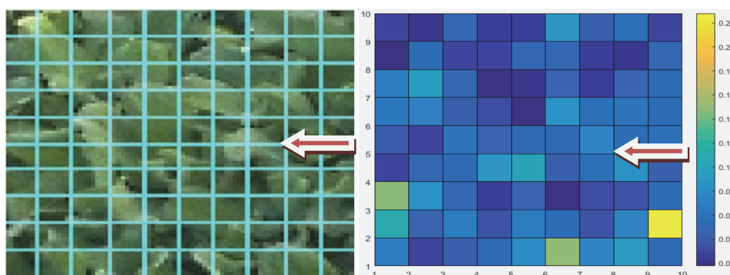
Рис. 4. Вид массива ПР, функционирующего в ЕМБП 02.10.2016 года. Слева – необработанное изображение, справа – обработанное и шкала условных цветов, обозначающих величину среднего квадратичного отклонения значения индекса С. Направление движения воды в ЕМБП справа-налево
