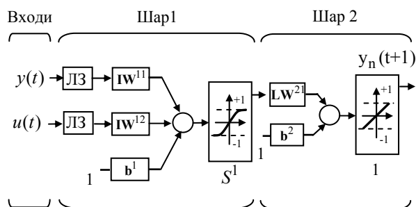
Рис. 2. Нейронна мережа регулятора керованого об'єкта
