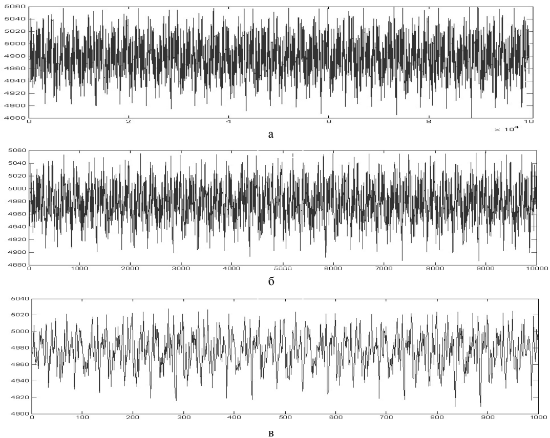
Рис. 2. Модель трафіку на основі ансамблю квазіперіодичних джерел з блоками агрегування m : а – m = 1 ; б – m = 10 ; в – m = 100
