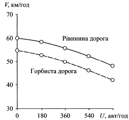
Рис. 2. Залежність середньої швидкості руху автопоїздів від інтенсивності руху для двосмугових доріг: рівнинна дорога ( \Pi = 6\% ), горбиста дорога ( \Pi = 40\% )
