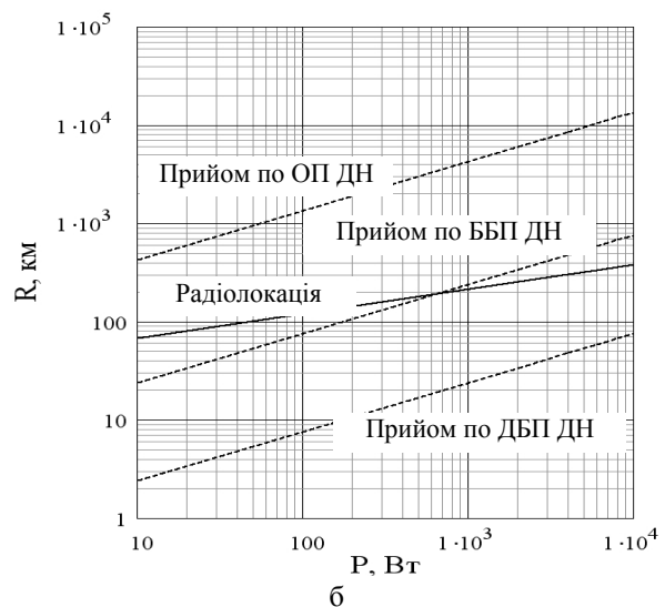
Рис. 2. Порівняння дальностей локації та прийому сигналу, що заважає, при випромінюванні останнього: а – за близькими; б – та далекими бічними пелюстками
