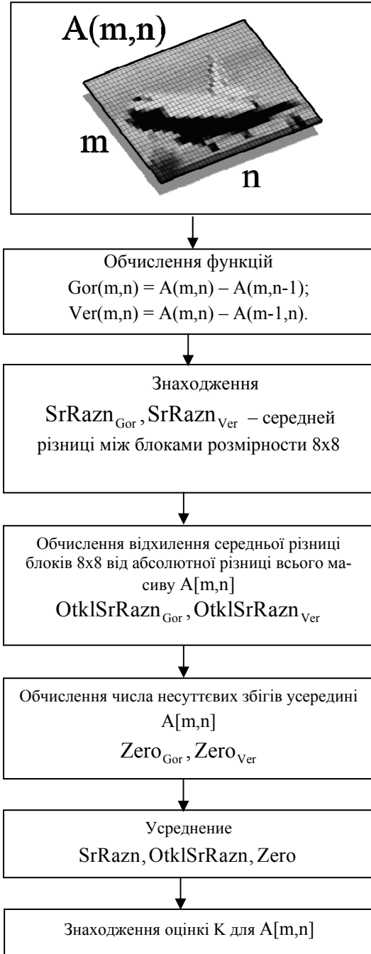
Рис. 1. Алгоритм оцінки якості зображення
