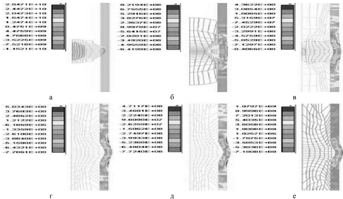
Рис. 2. Процес деформації сталюого циліндра товщиною 20 мм: а – t=1,449\text{E-}5\text{ с} ; б – t=4,199\text{E-}5\text{ с} ; в – t=7,199\text{E-}5\text{ с} ; г – t=1,095\text{E-}4\text{ с} ; д – t=1,169\text{E-}4\text{ с} ; е – t=1,39\text{E-}4\text{ с} (цифри – напруження в Па)
