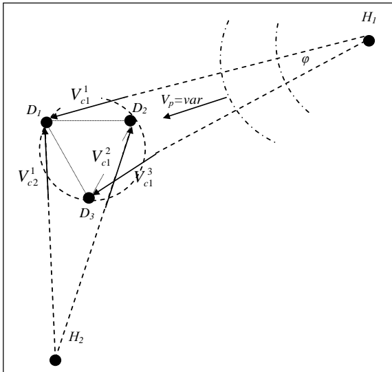
Рис. 1. Швидкість розповсюдження сейсмічної хвилі у зоні розміщення СП: V_{c1}^1, V_{c1}^3 – скаляр швидкості сейсмохвилі у напрямку від точки H_1 і до точок D_1, D_3 відповідно; V_{c2}^1, V_{c2}^2 – скаляр швидкості сейсмохвилі у напрямку від точки H_2 і до точок D_1, D_2 відповідно.
