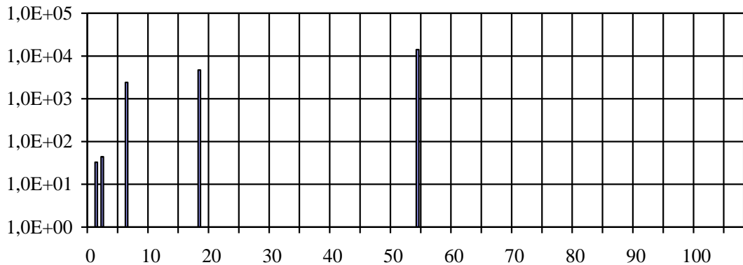
Рис. 2. Розподіл кількості ключів по довжинам періодів формованих послідовностей (експеримент 2, L_{\max} = 21352 )
