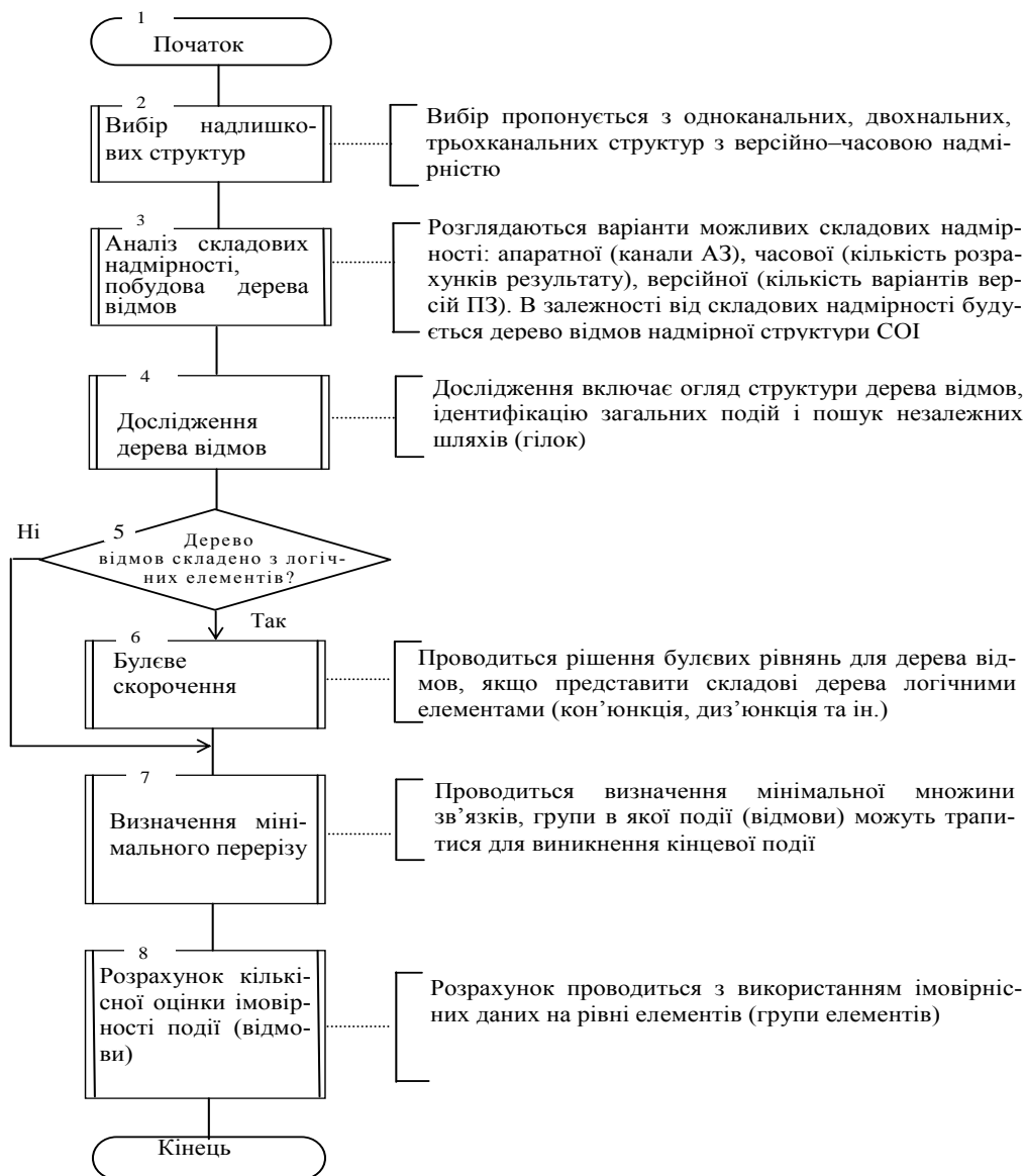
Рис. 4. Алгоритми проведення аналізу дерева відмов багатоканальних структур з версійно-часовою надмірністю
