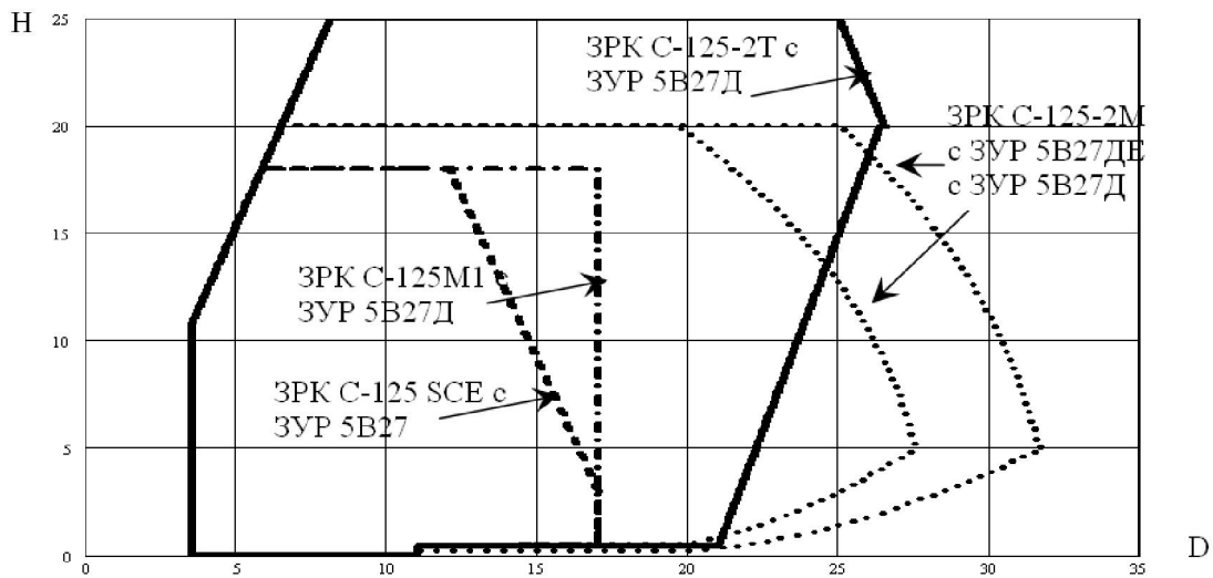
Рис. 1. Зоны поражения для различных вариантов модернизации ЗРК
