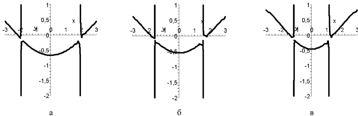
Рис. 2. Графіки зміни координати точки перетину осі OY лінією пеленга в залежності від віддаленості об'єкта від центра системи координат для різної топології тріади датчиків: база 2a = 2 м; лінією можливого місцеположення об'єкта є коло із радіусом 3a ; а – прямокутна рівнобедренна топологія датчиків; б – рівнобедренна топологія датчиків; в – рівностороння топологія датчиків
