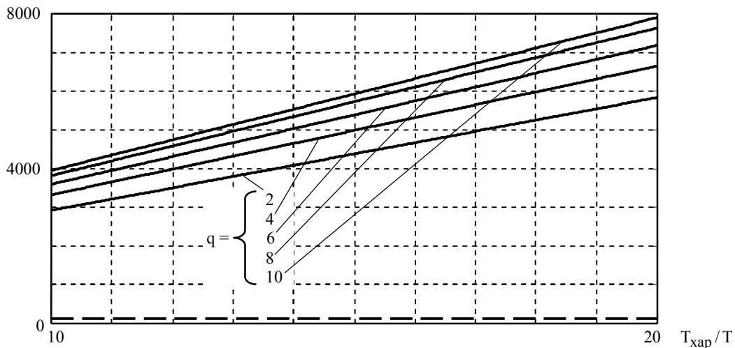
Рис. 1. Залежності оцінки параметра \sqrt{V_f} = \sigma_f від відношення T_{\text{хар}}/T : — початкова згідно (2); — запропонована в роботі [4] згідно (3) при різних значеннях q
