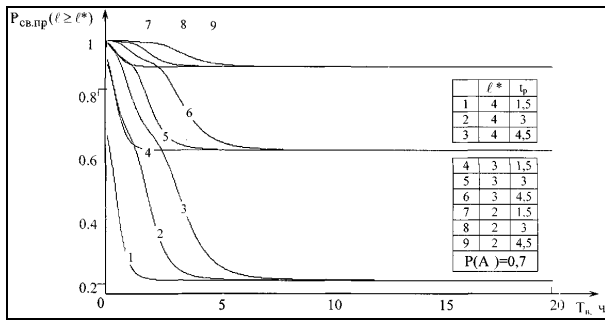
Рис. 3. Графіки залежностей величини P_{св.пр.}(l \ge l^*) для групи з чотирьох ЗРК від величини T_{п.ч} , при t_{в} \sim N(T_{в}, \sigma_{в}) , \sigma_{в} = 0,2T_{в} , t_{д} \sim N(T_{д} = 1 \text{ ч}, \sigma_{д} = 0,16 \text{ ч}) , P(A) = 0,7
