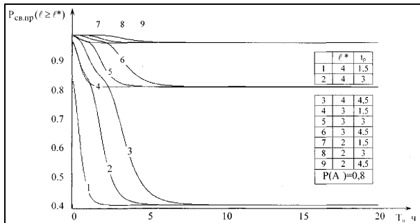
Рис. 4. Графіки залежностей величини P_{св.пр.}(l \ge l^*) для групи з чотирьох ЗРК від величини T_{п.ч} , при t_{в} \sim N(T_{в}, \sigma_{в}) , \sigma_{в} = 0,2T_{в} , t_{д} \sim N(T_{д} = 1 \text{ ч}, \sigma_{д} = 0,16 \text{ ч}) , P(A) = 0,8
