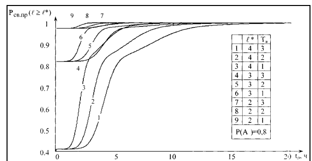
Рис. 2. Графіки залежностей величини P_{св.пр.}(l \geq l^*) для групи з чотирьох ЗРК від величини часу t_p , при t_B \sim N(T_B, \sigma_B), \sigma_B = 0,2T_B, t_D \sim N(T_D = 1 \text{ ч}, \sigma_B = 0,16 \text{ ч}), P(A) = 0,8
