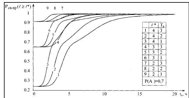
Рис. 1. Графіки залежностей величини P_{св.пр.}(l \geq l^*) для групи з чотирьох ЗРК від величини часу t_p , при t_B \sim N(T_B, \sigma_B), \sigma_B = 0,2T_B, t_D \sim N(T_D = 1 \text{ ч}, \sigma_B = 0,16 \text{ ч}), P(A) = 0,7
