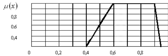
Рис. 3. Функція належності нечіткої ймовірності P_{\text{но}}
