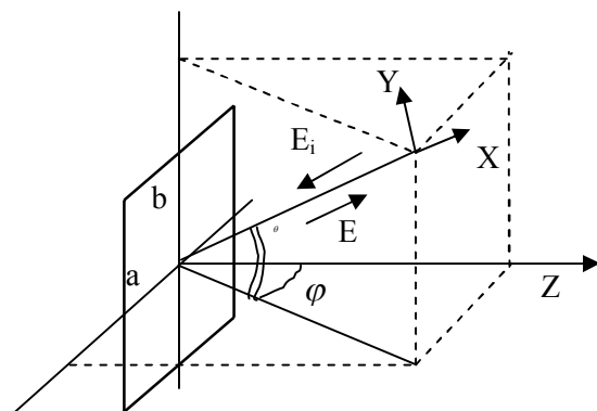
Рис. 2. Моностабичне розсіяння плоскої хвилі на прямокутній пластині
