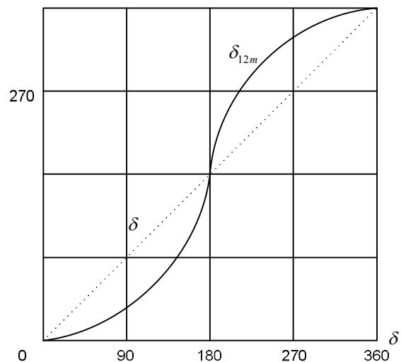
Рис. 3. Графік залежності \delta_{12m} від \delta
