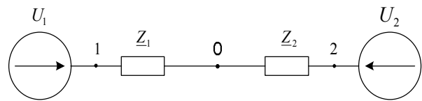
Рис. 1. Схема заміщення електропередачі
