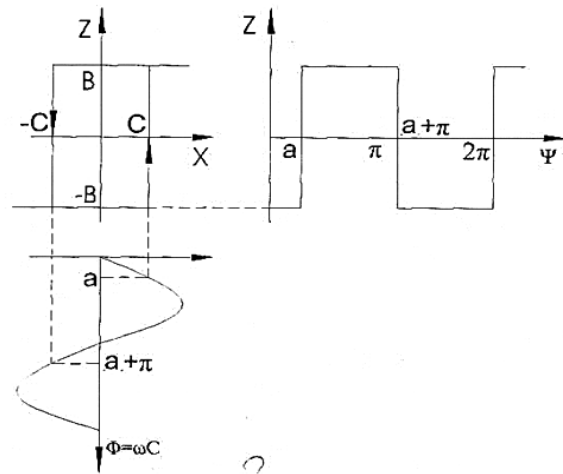
Рис. 2. Амплітудно-фазова характеристика нелінійного елемента
