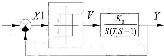
Рис. 1. Структурна схема моделювання нелінійності
