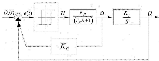
Рис. 4. Схема моделювання ДПС із релейним керуванням
