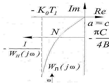
Рис. 3. Розрахунок стійкості і параметрів автоколивань
