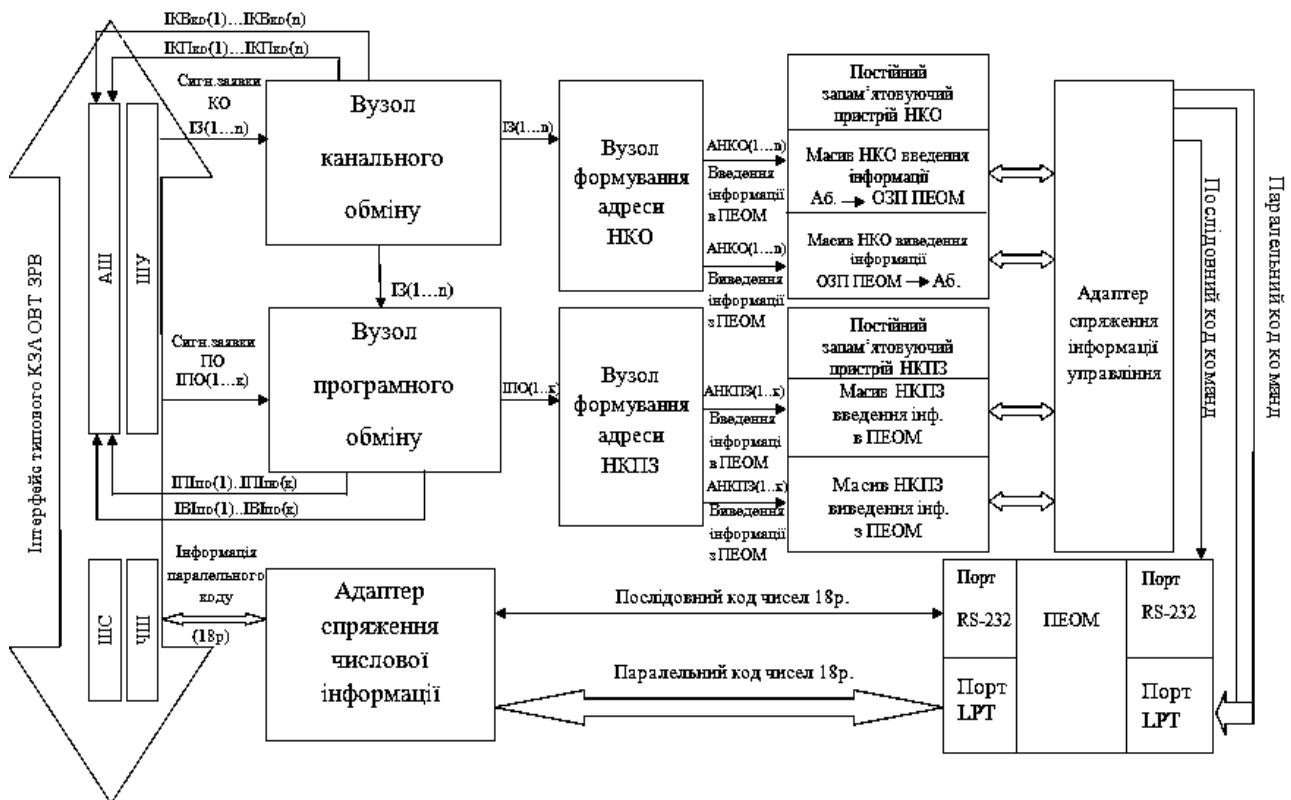
Рис. 1. Структурна схема пристрою інформаційного спряження ПЕОМ та типового інтерфейсу КЗА ОБТ ЗРВ
