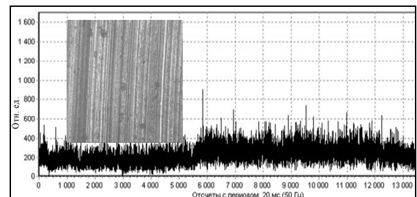
Рис. 4. Характер изменения спектральной мощности АЭ при моделировании повреждения трибосистем: распределительный золотник – торец ротора
